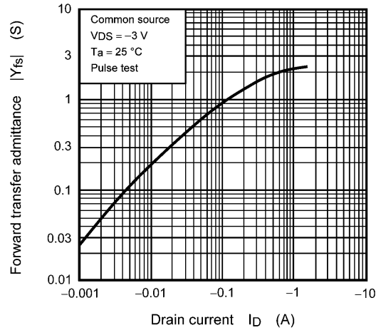
Fig. 8.8 |Y_{fs}| - I_D
