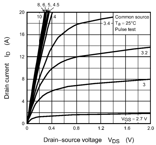
Fig. 8.2.2 I_D - V_{DS}
