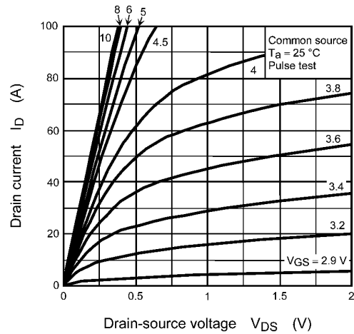
Fig. 8.2 I_D - V_{DS}
