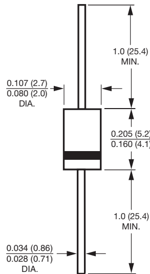
DO-204AL (DO-41)
